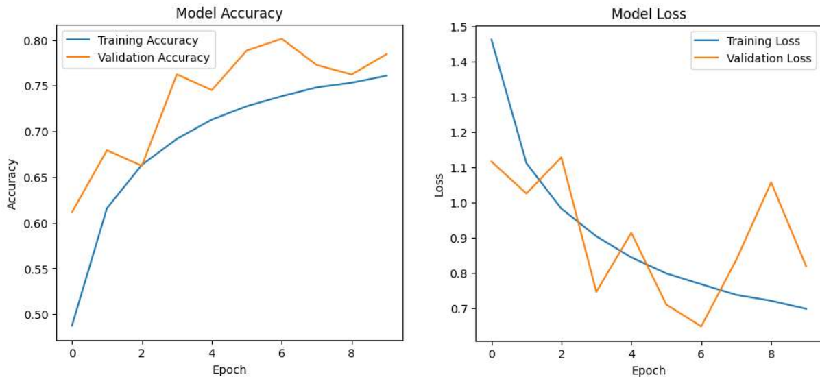
Gambar 2. Perubahan accuracy dan loss selama pelatihan
